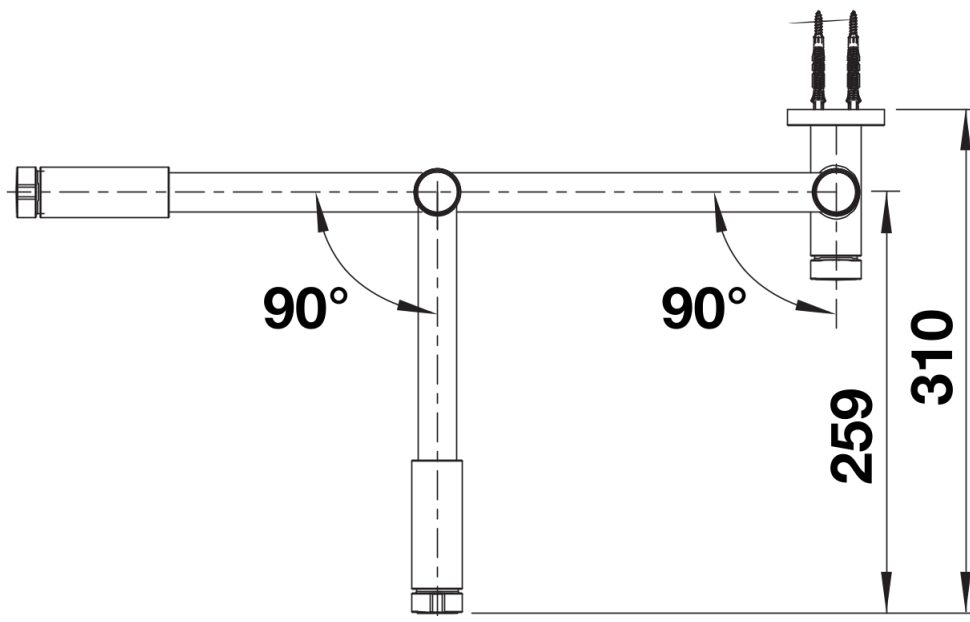
Swivel range
