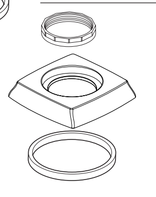
RP77196▲ Handle Base, Nut & Gasket Base de la Manija, Tuerca y Empaque Base, écrou et joint de manette
