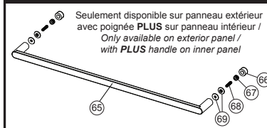
Barre à serviette / Towel bar 104484-XXX **
