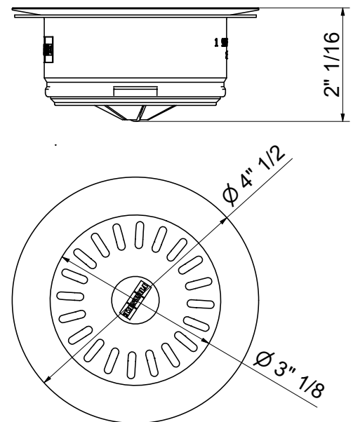
Dessin coté
