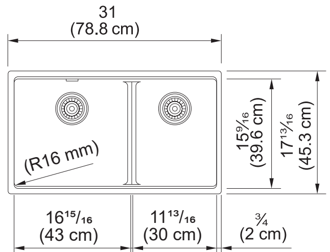
Dessin coté
