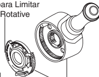
RP72567 ▲ Handle Assembly Ensemble de la Manija Poignée
