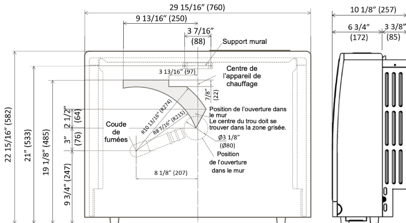
Vue avant (avec exemple de gabarit mural sur l'emballage en carton de l'appareil)
