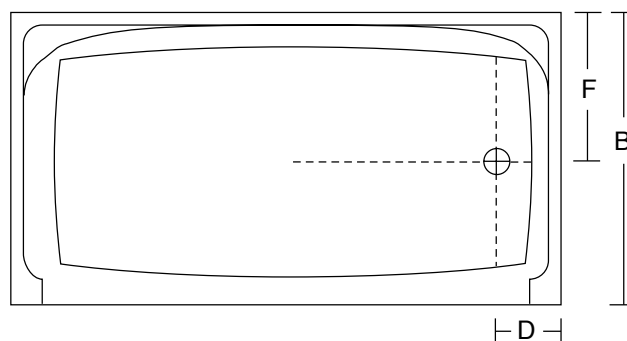
Top View R.H. Model
